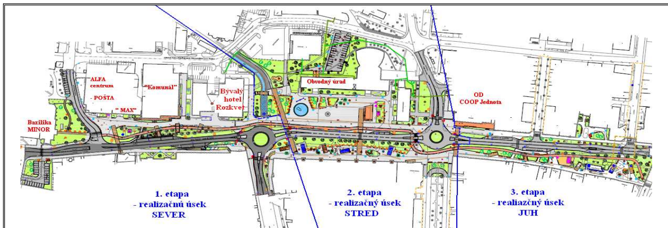
Obr. č.1: Úprava centra mesta Vranov nad Topľou – rozdelenie realizácie na realizačné úseky
